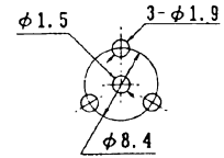
取り付け穴寸法
