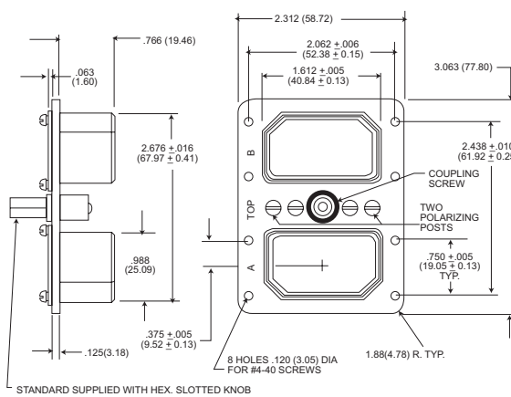
DPX2-33M (Male)
