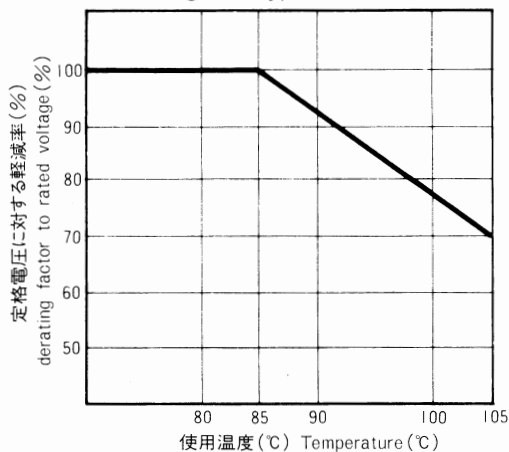
グラフ② 適用Type MMH (63V)
