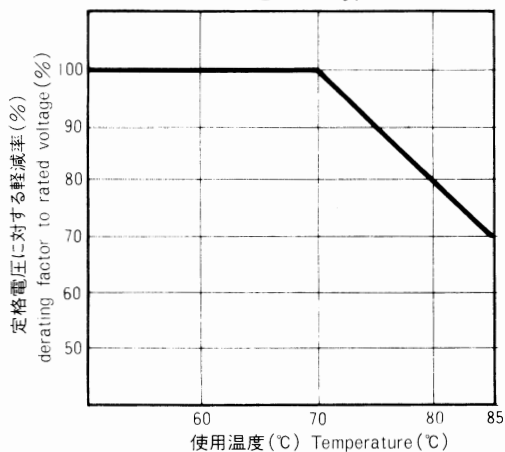
グラフ① 適用Type APS.APH
