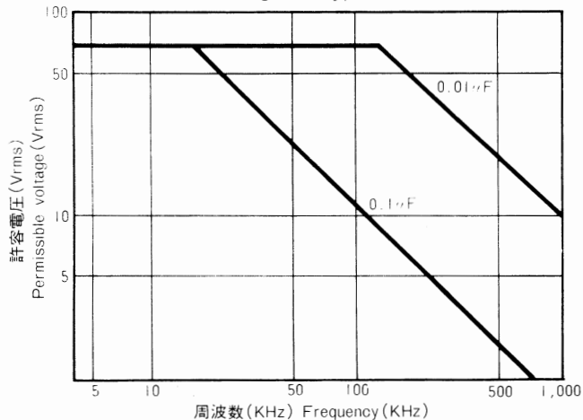
グラフ① 適用Type APS
