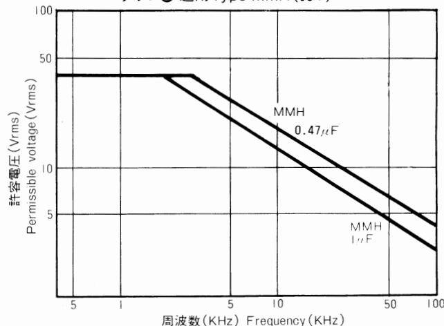
グラフ② 適用Type MMH (63V)
