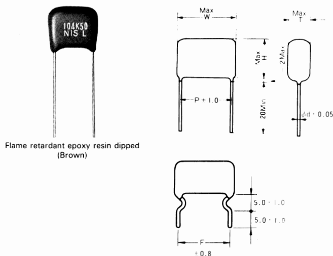
シングルフォーミング / Single Forming
