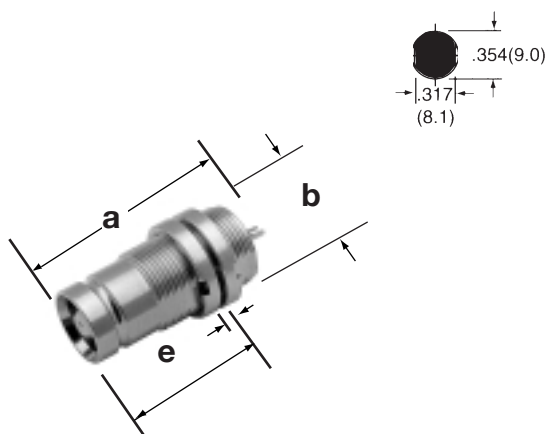
Receptacle 156-343-03
