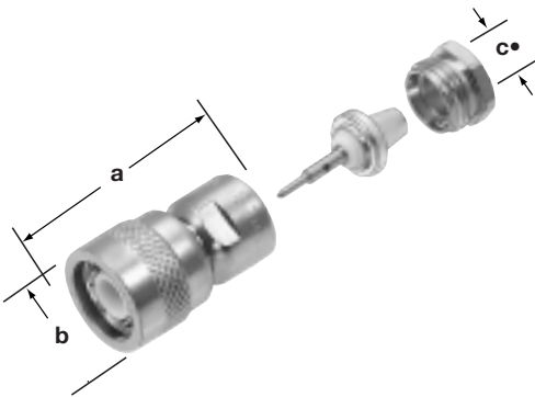
TNC QUICKTRIM® Plug 31-5061
