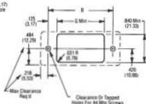
26-4401-30XS or 26-4401-30XP Receptacle
