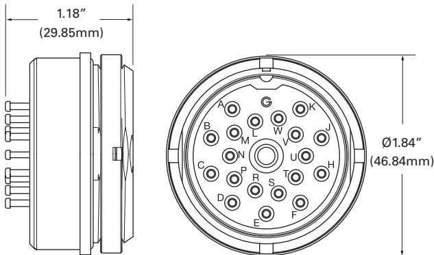
UW2026FD00 receptacle
