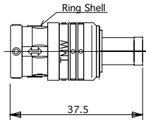
BNCS705-P(°)
