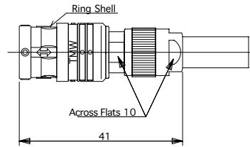
BNCS710-P(°)
