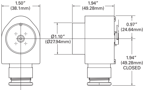
UW 1320 plug
