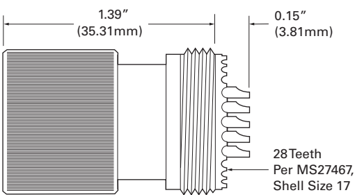
19-Contact CIA3245089-3
