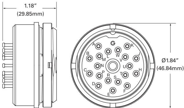
UW2026FD00 receptacle
