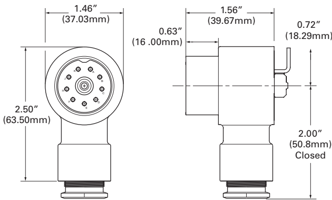
UW 1220 plug
