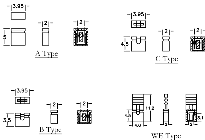
2106-Series 2.0mm(0.079")
