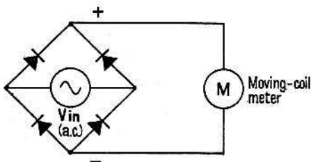
Fig. 2 Meter Rectifier.
