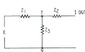
Fig. 13a. T attenuator
