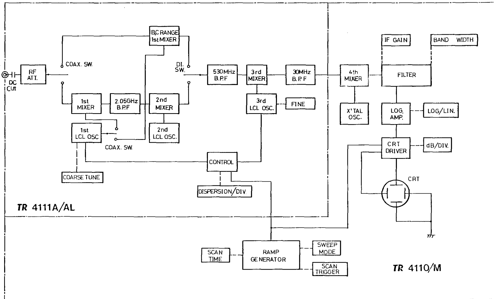
図 3-1 TR 4110/M, TR 4111AL ブロック図
