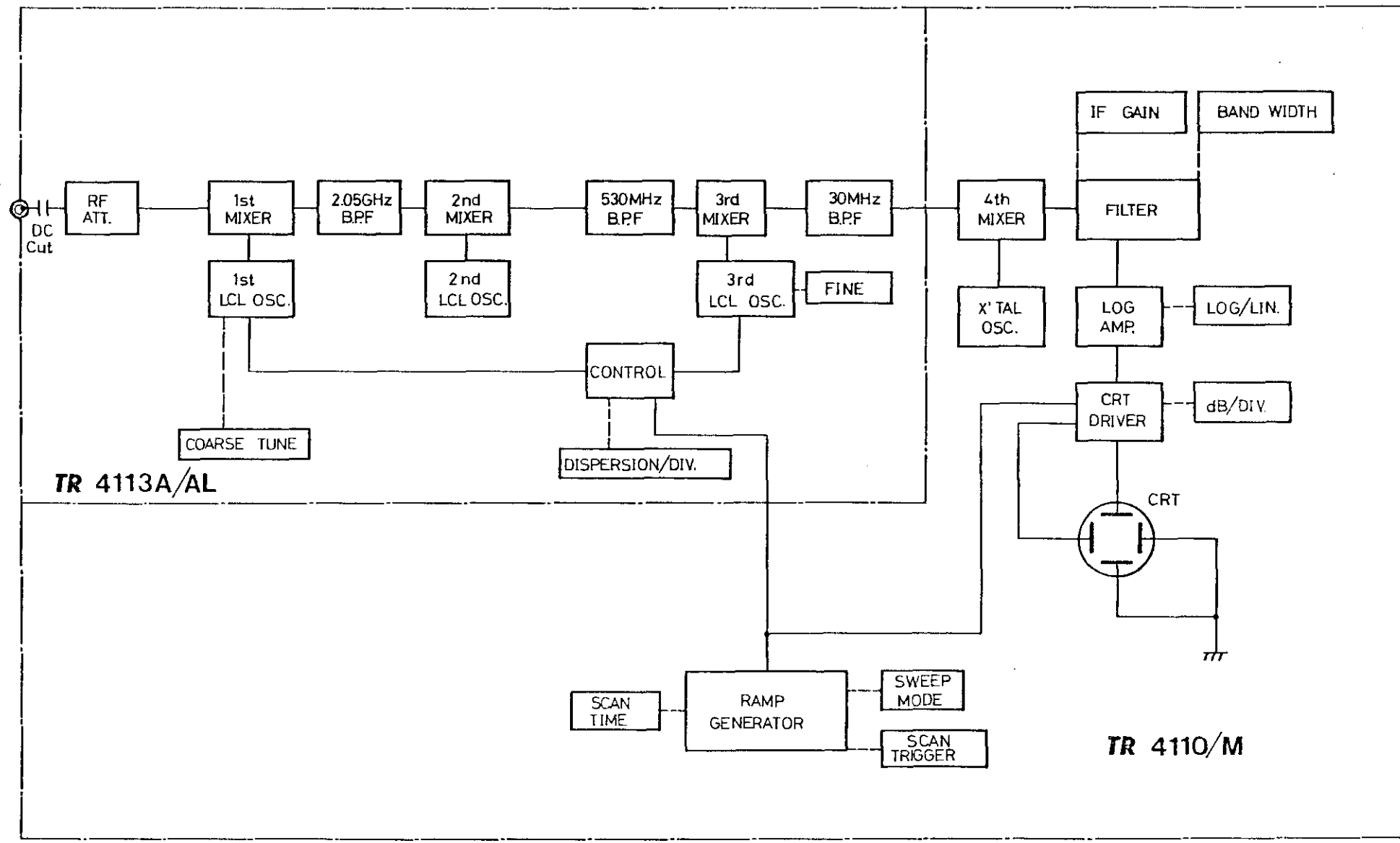
図 3-2 TR 4110/M, TR 4113AL ブロック図
