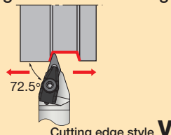
Cutting edge style V
