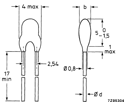
Fig. 1 0,1 W types.
