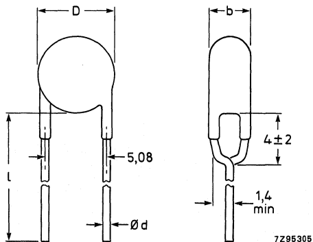
Fig. 2 0,25 and 0,75 W types.
