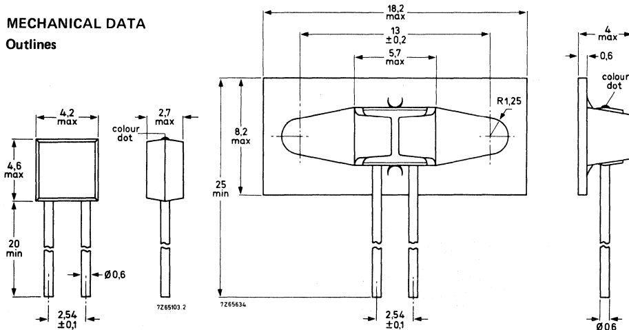
type 2322 640 90004
