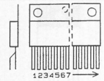
QILP
