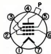
7BM
