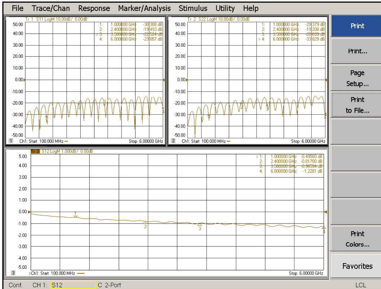
21N-21N-RG316-0M35-Test
