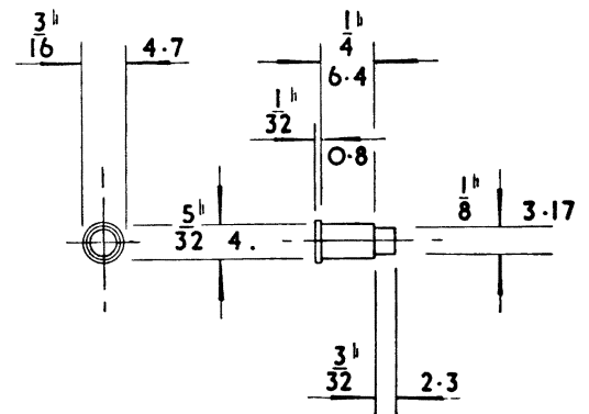
1/2" DIA. PULLEY PIVOT.
