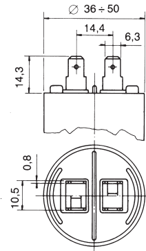
Fig. 1 Doppio Faston 6,35 x 0,8 mm
