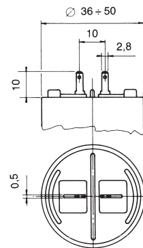
Fig. 3 Faston 2,8 x 0,5 mm
