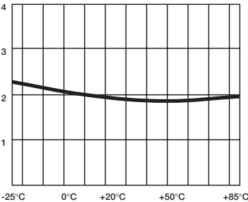
Angolo di perdita Dissipation factor
