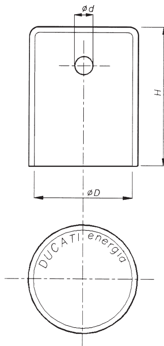
Fig. 8 Cappellotto. Fig. 8 Protective cap.
