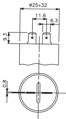
Fig. 2 Faston semplice 6,3 x 0,8 mm
