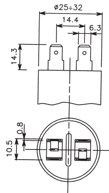
Fig. 1 Doppio Faston 6,35 x 0,8 mm
