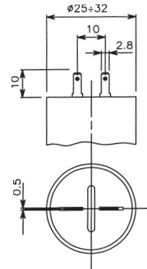
Fig. 3 Faston 2,8 x 0,5 mm
