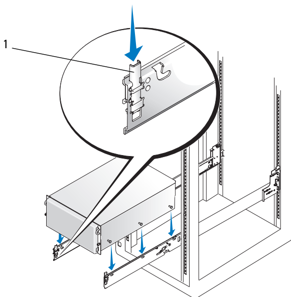
Figure 1-7. Installation du système dans le rack
