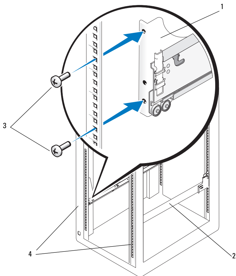
Ilustración 1-6. Montaje de los ensamblajes de rieles VersaRails
