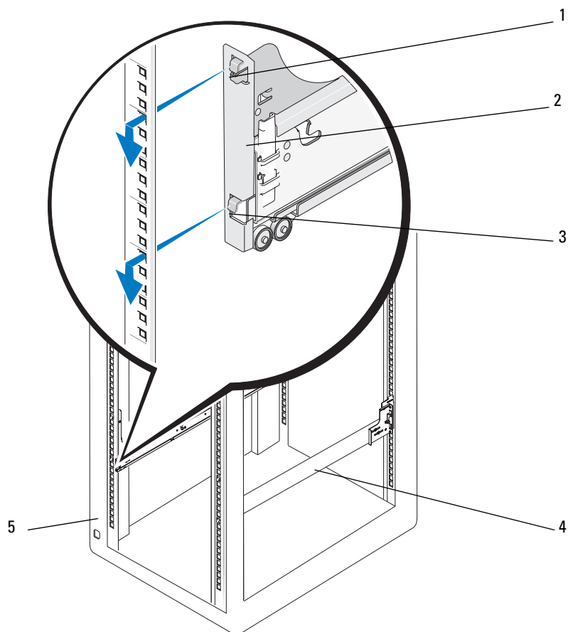
Figure 1-5. Installation des assemblages à glissière RapidRails
