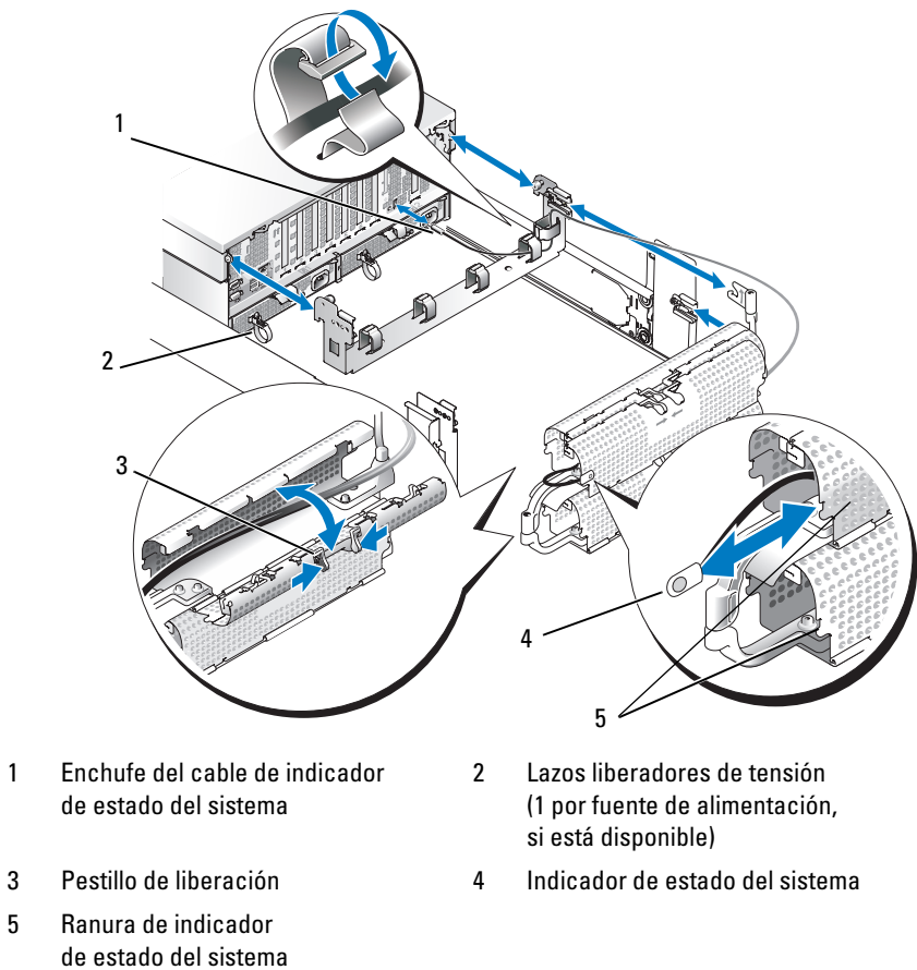
Ilustración 1-9. Instalación del cable de indicador de estado del sistema
