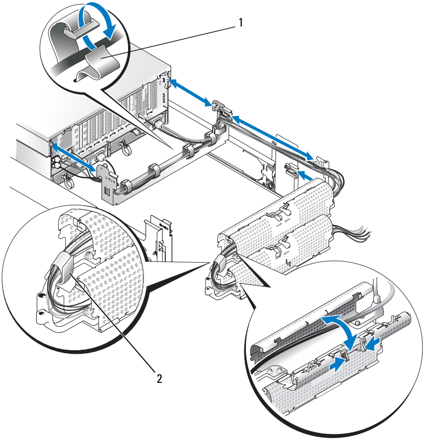
Ilustración 1-10. Cableado en el brazo para tendido de cables
