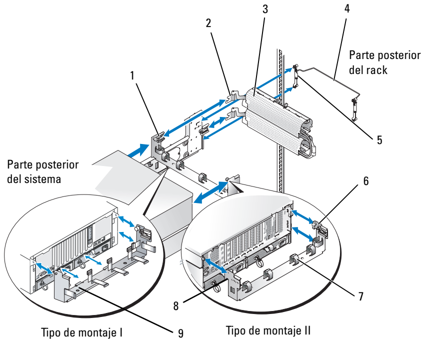
Ilustración 1-8. Instalación del brazo para tendido de cables
