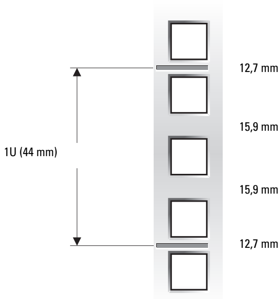
Abbildung 1-3. Eine Rack-Einheit
