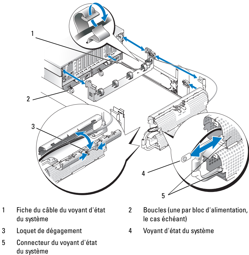
Figure 1-9. Installation du câble du voyant d'état du système
