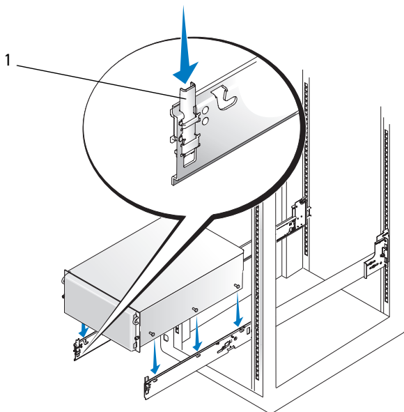
Figure 1-7. Installation du système dans le rack
