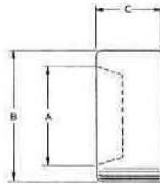
Fig. 39. Conduit ferrule Type G
