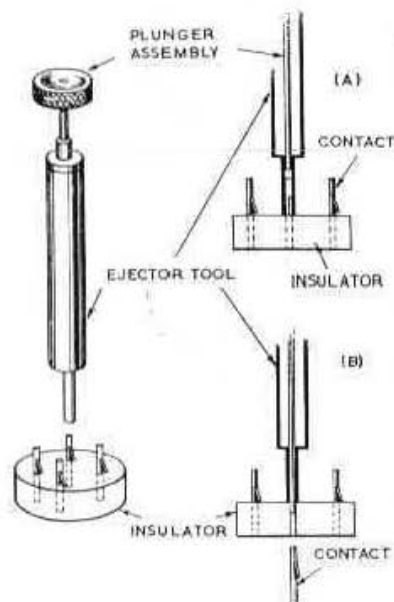
Fig. 19. Ejector tool
