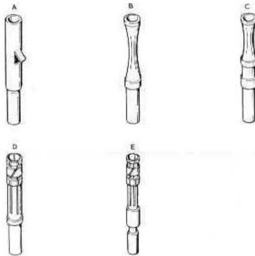
Fig. 21. Contacts
