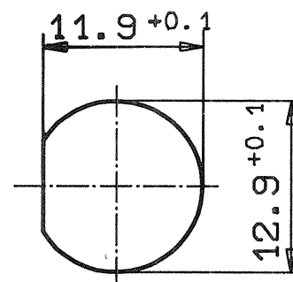
MONTAGEBOHRUNG
