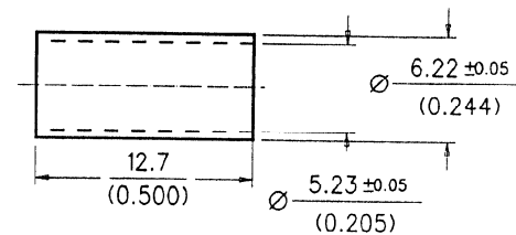
FERRULE
