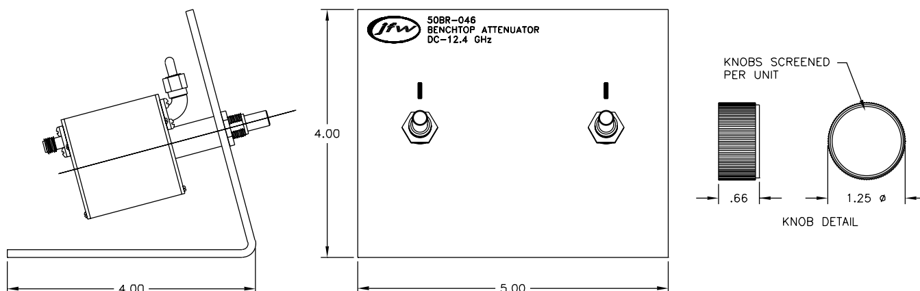
50BR-046
