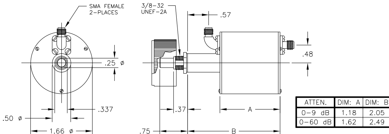
50BR-046
