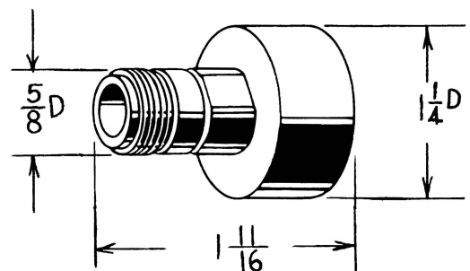
JACK — 50 ohm
