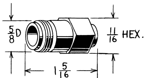
JACK — 50 ohm
