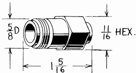
JACK — 50 ohm
