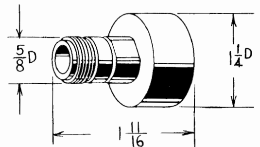
JACK — 50 ohm
