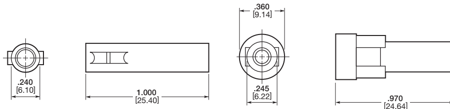
Receptacle
