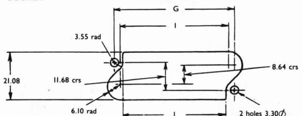
Socket
