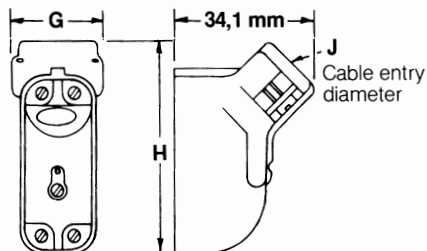
Cable outlet
