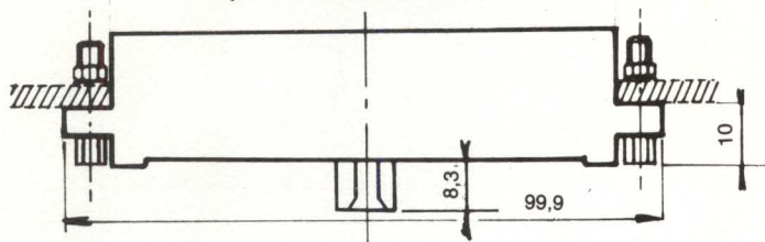
Isolant spécial embase «SPL» Special socket insulator «SPL»
