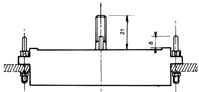
Isolant spécial fiche «SPL» Special plug insulator «SPL»
