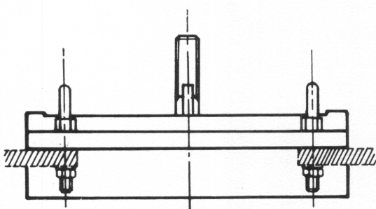
Isolant fiche — Plug insulator
