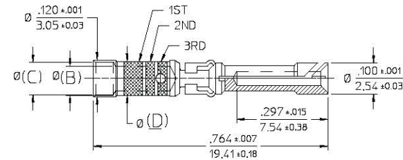
CATALOG NO M39029/35-274 SHOWN
