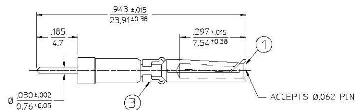
CATALOG NO 8125-Δ SHOWN
