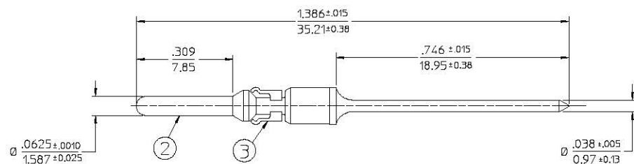
CATALOG NO 7130 SHOWN
