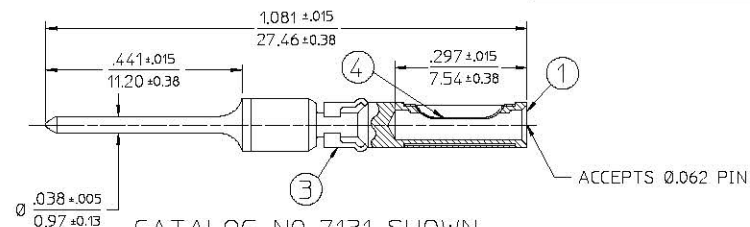
CATALOG NO 7131 SHOWN
