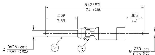
CATALOG NO 8124-Δ SHOWN
