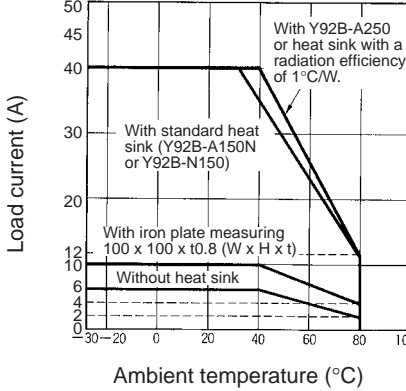
G3NA-440B
