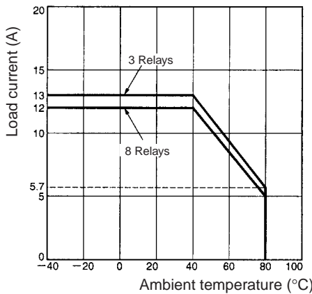
G3PB-235B-VD
