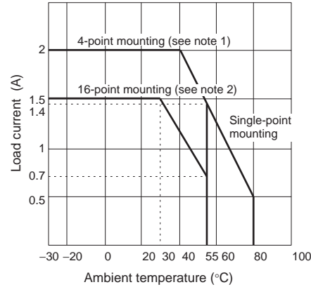
G3R-OA202SZN-UTU/OA202SLN-UTU
