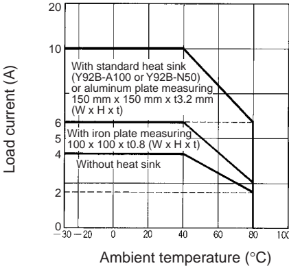
G3NA-D210B
