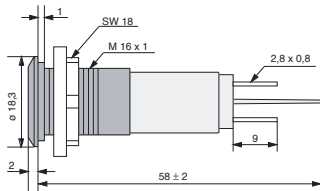
Kunststoffausführung / version with black plastic bezel
