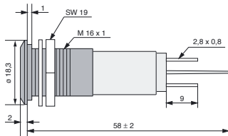
Metallausführung / version with metal bezel
