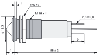
Metallausführung / version with metal bezel
