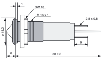
Kunststoffausführung / version with black plastic bezel
