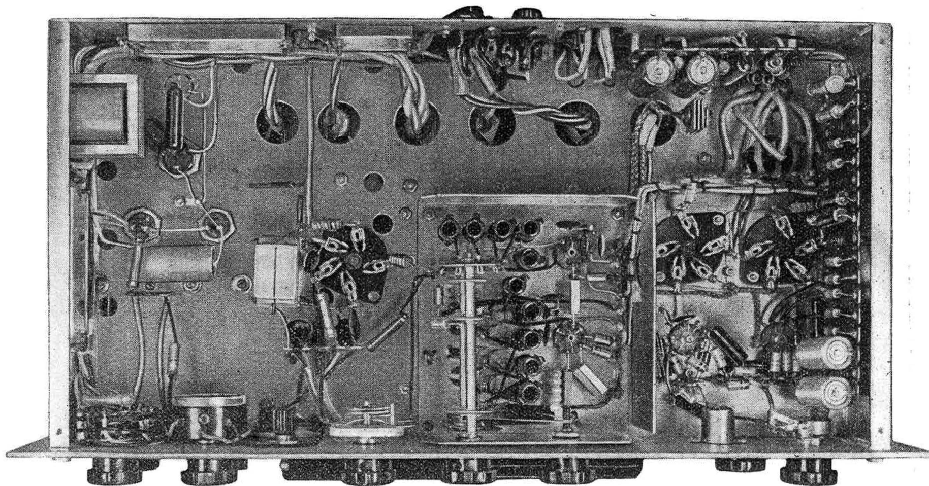
G 212-TR - Vista degli organi e dei collegamenti posti sotto al telaio.
