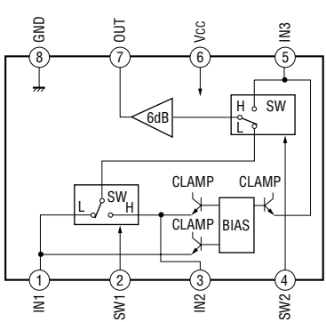
MM1228XFBE (IC101)
