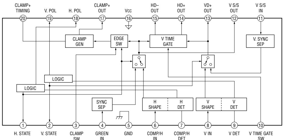
M52347FP-TE (IC303)
