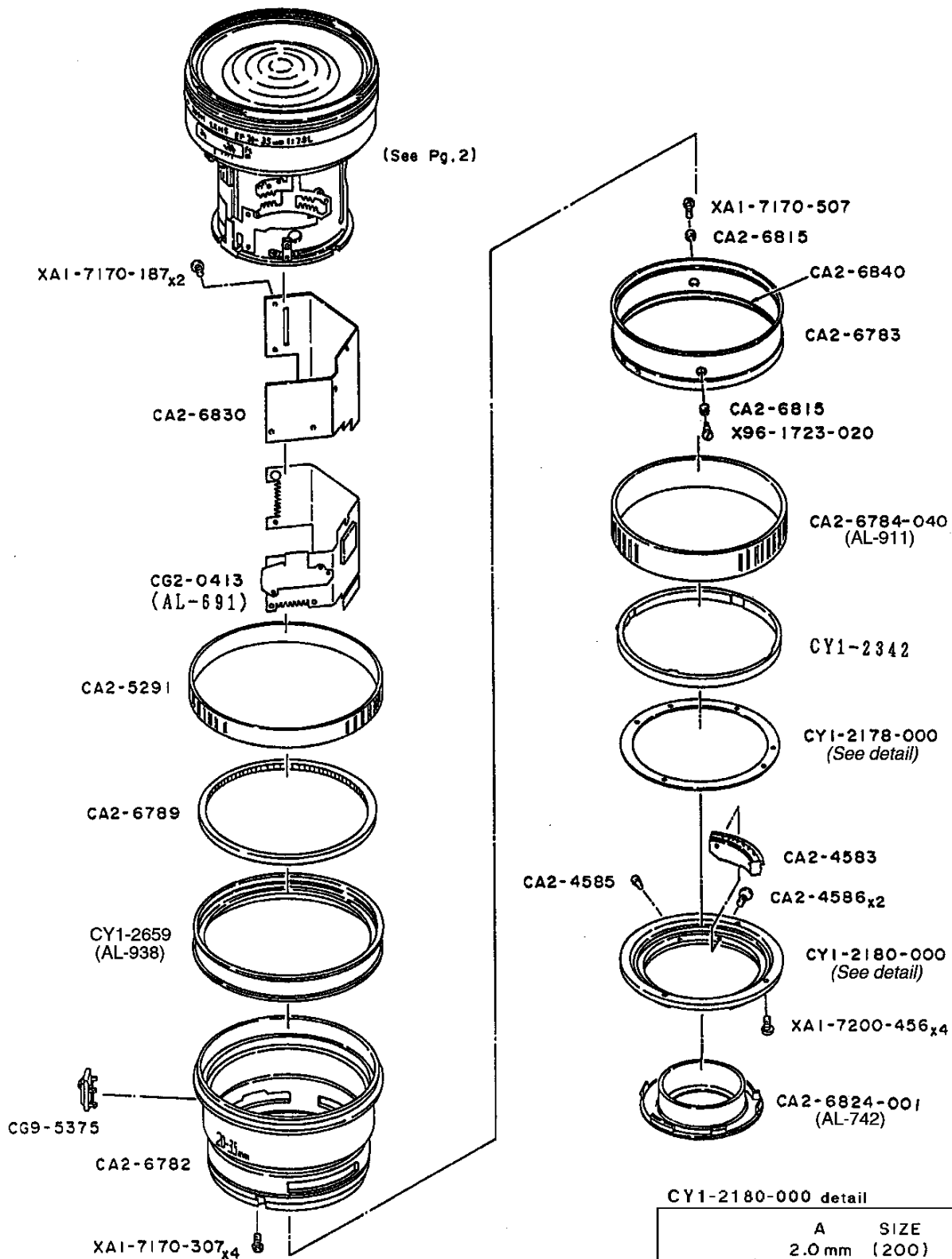
CY1-2178-000 detail
