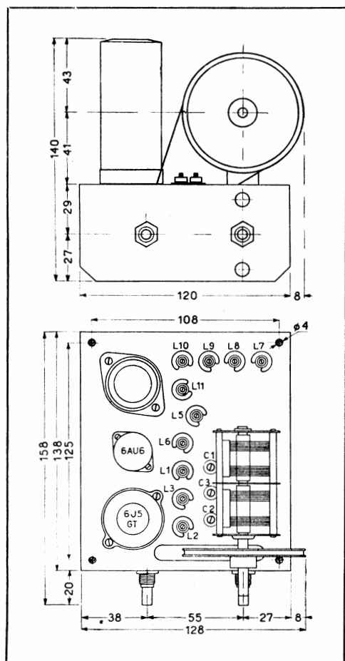
Dati di ingombro e disposizione delle valvole, delle induttanze e delle viti di regolazione del Gruppo VFO tipo 4/101. Il Gruppo VFO 4/102 ha la medesima disposizione e lo stesso ingombro, eccetto la dimensione verticale sopra il piano del telaio che, a causa della valvola 6L6, è maggiore.
