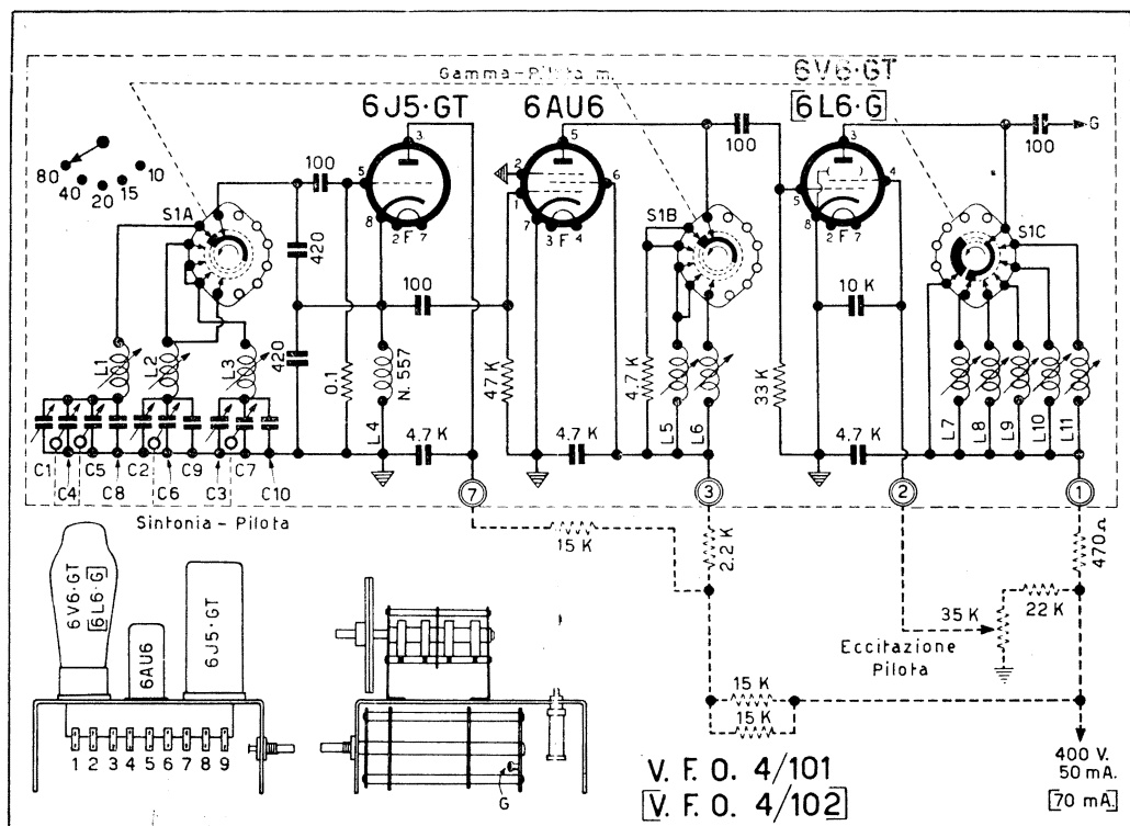
Schema elettrico dei Gruppi VFO n. 4/101 e n. 4/102
