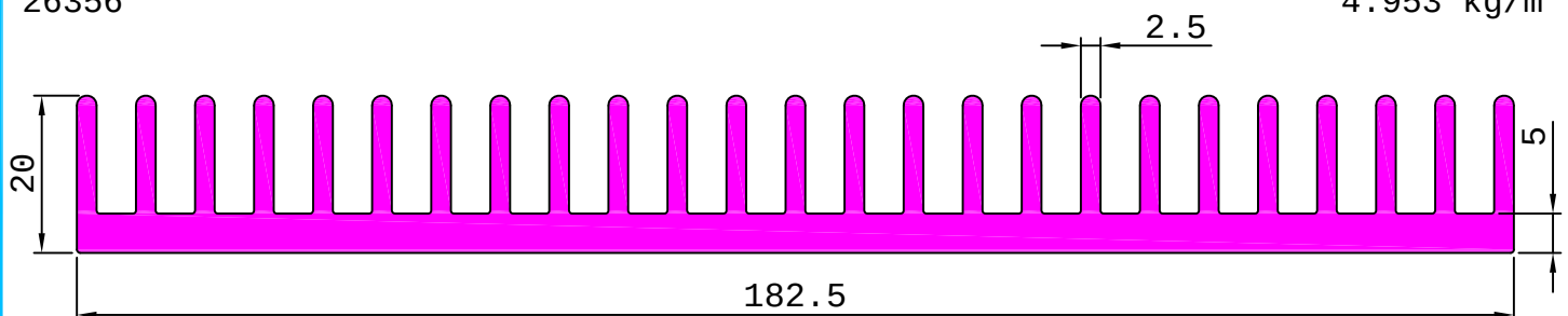
26356 4.953 kg/m
