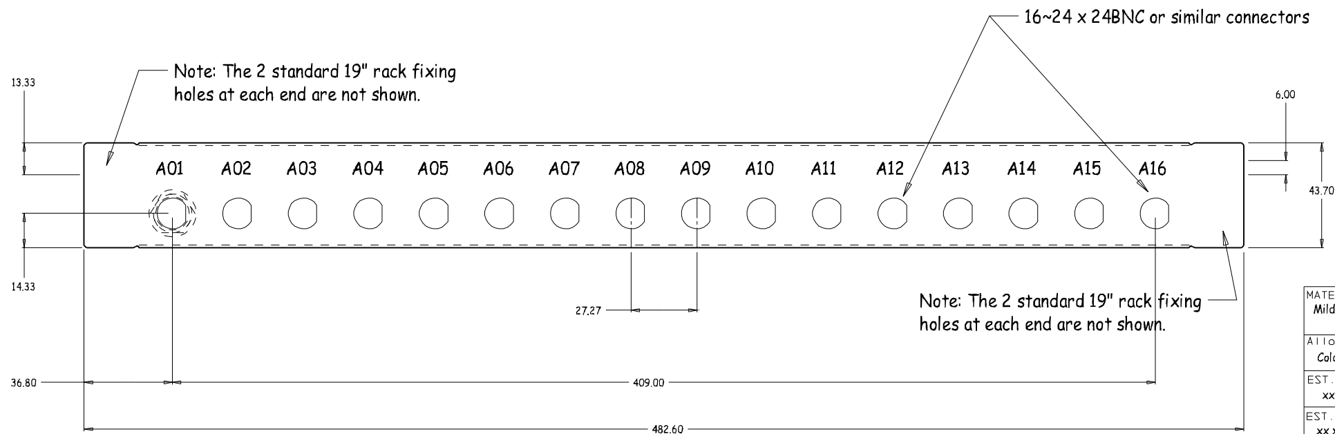
CASA Drawing: PP1U-24x24BNC-MS12
